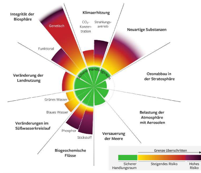
Abb. 2: Konzept der planetaren Grenzen; Quelle Richardson et al.: Earth beyond six of nine planetary boundaries. In: Science Advances. September 2023
